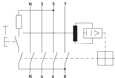
Anschlusschema
