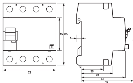
Maßzeichnung Fehlerstromschutzschalter DFS 4 125-4/0,30-A HD
