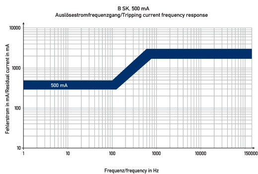
Diagramme Fehlerstromschutzschalter DFS 4 125-4/0,50-B SK HD
