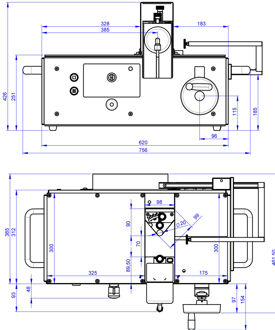
Kuva 2: Mitat
