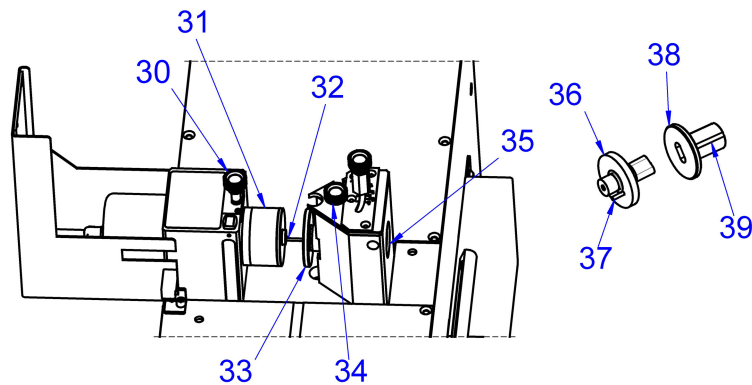
Kuva 7: Virtakiskon lävistäminen
