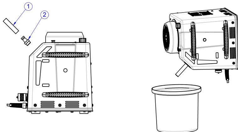
Kuva 6: Öljynvaihto
