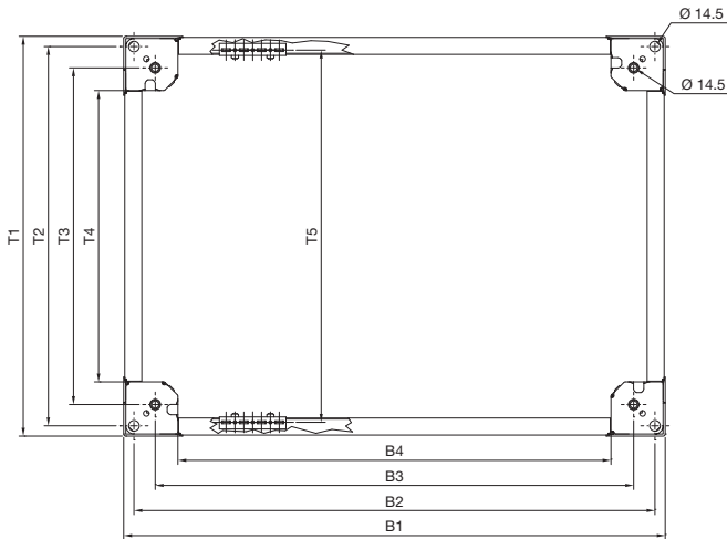
Sokkel, 100 mm høj
