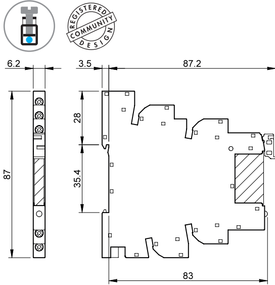
Typ 39.10/39.20 39.11/39.21 Schraubklemmen
