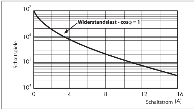
F 45 - Elektrische Lebensdauer bei AC Typ 45.31/45.91
