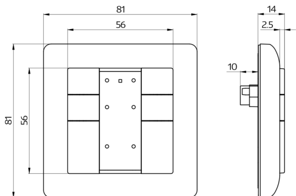
Bemaßung 93176
