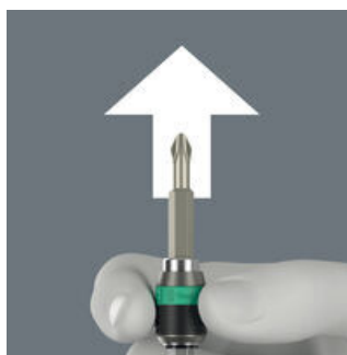
Zum Bitwechsel einfach die Hülse nach vorne schieben: Dabei hebt der Federmechanismus den Bit vom Magneten ab und entriegelt das Werkzeug. Der Bit kann problemlos entnommen werden. Besonders hilfreich: Mühelose Entnahme auch kleinster Bitgrößen ohne Hilfswerkzeug.
