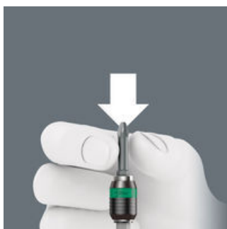
Ohne Betätigung der Hülse kann der Bit in die Aufnahme geschoben werden. Sobald der Bit in der Schraube angesetzt wird, wird die Verriegelung automatisch aktiviert. Der Bit sitzt sicher und wackelfrei.
