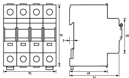
Maßzeichnung Lasttrennschalter RH o8o-4oo
