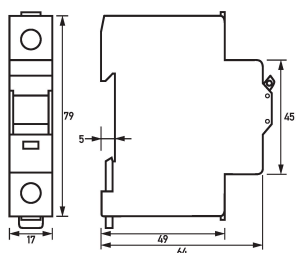
Maßzeichnung Gruppenansicht
