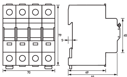
Maßzeichnung Gruppenansicht
