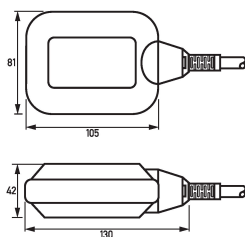
Maßzeichnung Schwimmerschalter Champ 2 GS-L/F 03 m
