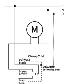
Schaltungsbeispiel Schwimmerschalter Champ 2 GS-L/F 03 m
