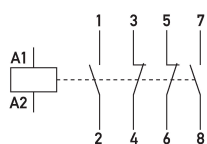
Schaltungsbeispiel Installationsschütze HS 2-230AC/25-22
