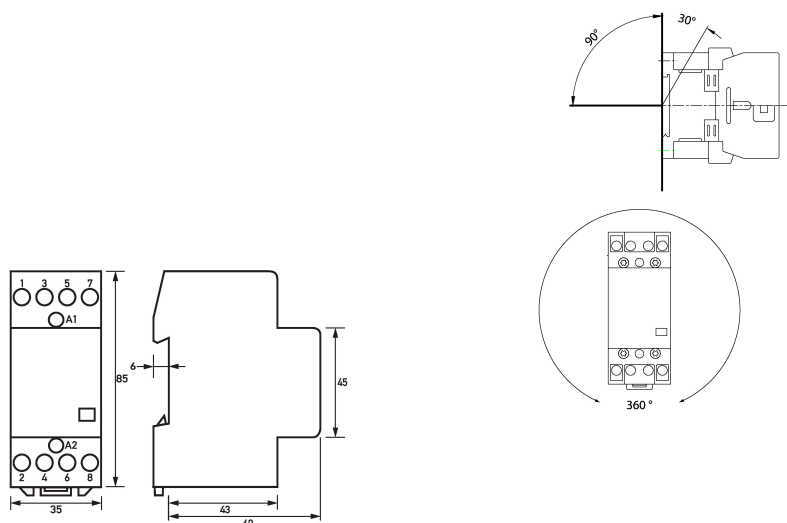
Maßzeichnung Installationsschütze HS 2-230AC/25-22
