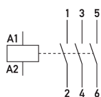
Schaltungsbeispiel Installationsschütze HS 2-230AC/25-30
