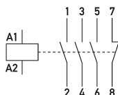
Schaltungsbeispiel Installationsschütze HS 2-230UC/25-31
