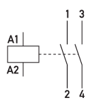
Schaltungsbeispiel Installationsschütze HS 1-230AC/25-20
