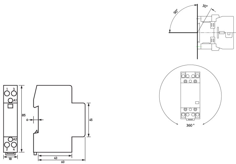
Maßzeichnung Installationsschütze HS 1-230AC/25-20
