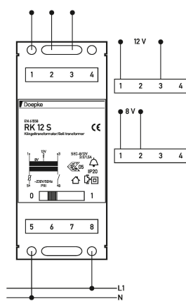
Schaltungsbeispiel Klingeltransformatoren RK 12 S
