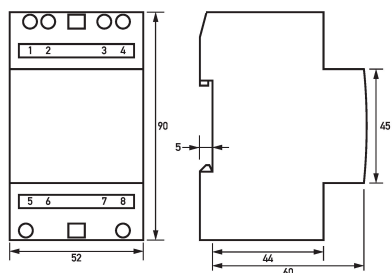
Maßzeichnung Gruppenansicht
