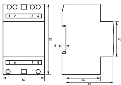
Maßzeichnung Klingeltransformatoren RK 3 U
