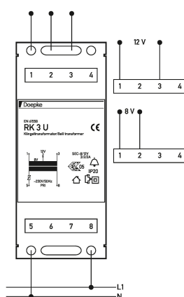
Schaltungsbeispiel Klingeltransformatoren RK 3 U
