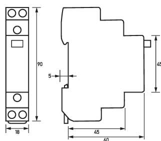
Maßzeichnung Steuerschalter RSS 016-200
