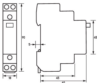
Maßzeichnung Steuerschalter RSS 016-200L
