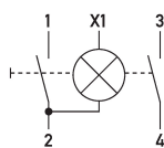
Schaltungsbeispiel Steuerschalter RSS 016-200L
