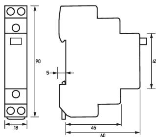
Maßzeichnung Stromstoßschalter (Fernschalter) RS 230-110
