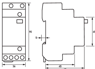
Maßzeichnung Gruppenansicht
