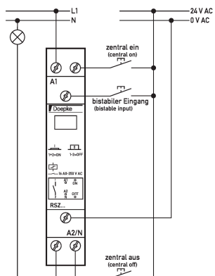
Schaltungsbeispiel Stromstoßschalter mit Zentralsteuerung RSZ 230-100
