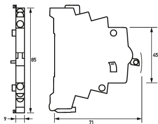
Maßzeichnung Hilfsschalter DHi 7
