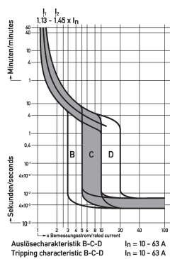
Diagramme Leitungsschutzschalter DLS 6h C13-1
