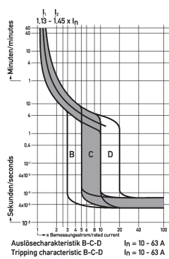
Diagramme Leitungsschutzschalter DLS 6i B20-1+N
