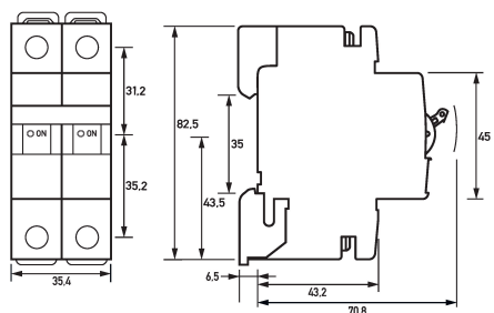
Maßzeichnung Leitungsschutzschalter DLS 6i B20-1+N
