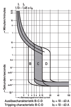
Diagramme Leitungsschutzschalter DLS 6i B50-2
