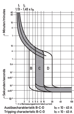
Diagramme Leitungsschutzschalter DLS 6i B32-4
