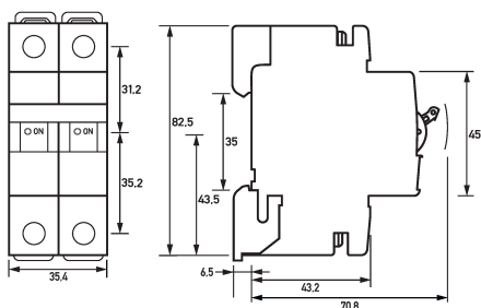
Maßzeichnung Leitungsschutzschalter DLS 6i D20-2
