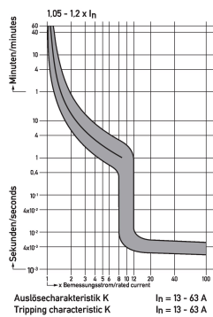
Diagramme Leitungsschutzschalter DLS 6i K32-3+N
