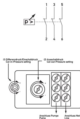
Anschlussschema
