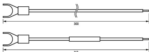
Maßzeichnung Kabel DFA 2 - RC 300
