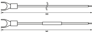
Maßzeichnung Gruppenansicht
