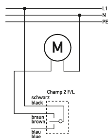
Schaltungsbeispiel Schwimmerschalter Champ 2 G-L/F HD 10 m
