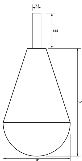
Maßzeichnung Schwimmerschalter Champ 2 G-L/F HD 10 m
