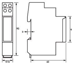
Maßzeichnung Gruppenansicht
