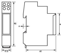
Maßzeichnung Gruppenansicht
