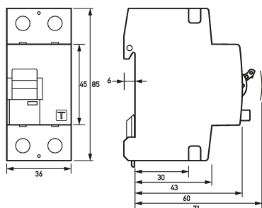
Maßzeichnung Gruppenansicht
