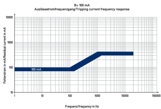
Diagramme Fehlerstromschutzschalter DFS 4 025-4/0,10-B+
