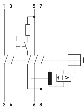
Schaltungsbeispiel Fehlerstromschutzschalter DFS 4W o63-2/0,50-A
