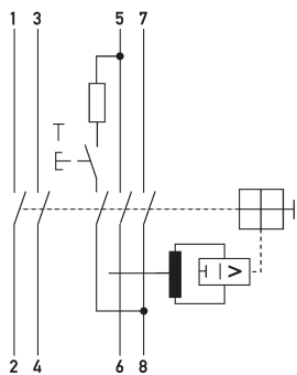
Schaltungsbeispiel Fehlerstromschutzschalter DFS 4W 063-2/0,50-A
