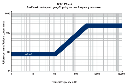
Diagramme Fehlerstromschutzschalter DFS 4 080-4/0,10-B SK V500
