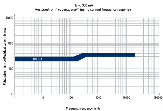
Diagramme Fehlerstromschutzschalter DFS 4 080-4/0,30-B+
