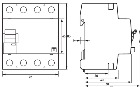
Maßzeichnung Fehlerstromschutzschalter DFS 4 080-4/0,30-B NK S
