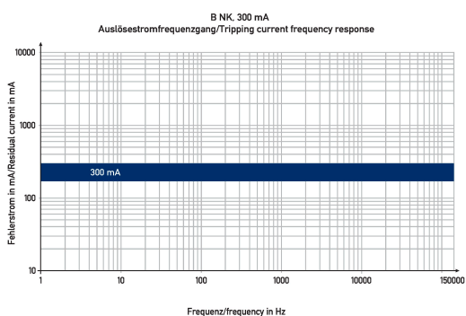
Diagramme Fehlerstromschutzschalter DFS 4 080-4/0,30-B NK S
