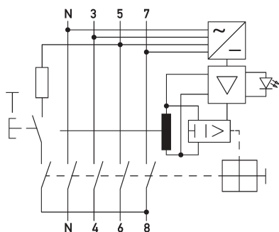
Schaltungsbeispiel Fehlerstromschutzschalter DFS 4 080-4/0,30-B NK S
