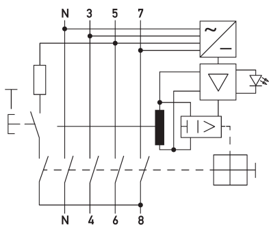
Schaltungsbeispiel Fehlerstromschutzschalter DFS 4 080-4/0,30-B NK
