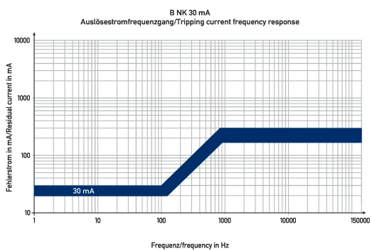
Diagramme Fehlerstromschutzschalter DFS 4 100-2/0,03-B NK
