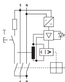
Schaltungsbeispiel Fehlerstromschutzschalter DFS 4 100-2/0,03-B NK
