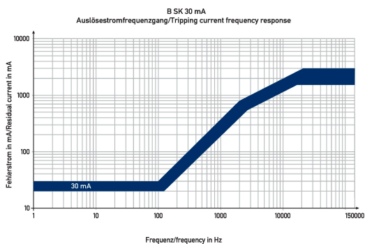
Diagramme Fehlerstromschutzschalter DFS 4 100-2/0,03-B SK
