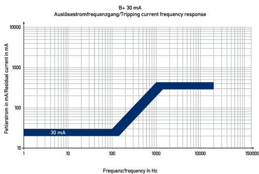
Diagramme Fehlerstromschutzschalter DFS 4 100-4/0,03-B+
