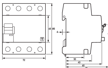
Maßzeichnung Fehlerstromschutzschalter DFS 4 100-4/0,03-A
