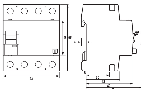
Maßzeichnung Fehlerstromschutzschalter DFS 4 100-4/0,03-A V500
