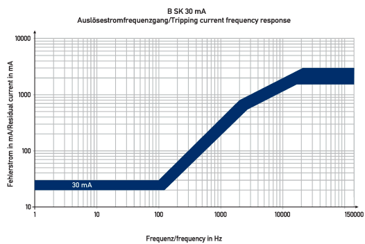
Diagramme Fehlerstromschutzschalter DFS 4 100-4/0,03-B SK V500
