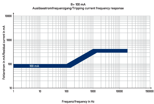
Diagramme Fehlerstromschutzschalter DFS 4 100-2/0,10-B+
